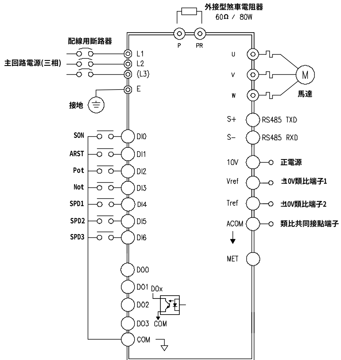
標準端子接線圖 - 速度控制模式
