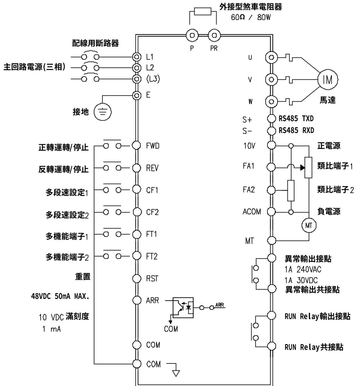
標準端子接線圖
