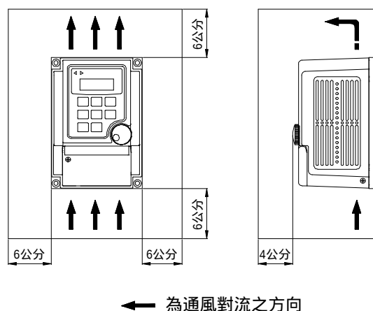
圖 6-1 安裝的方向與空間
